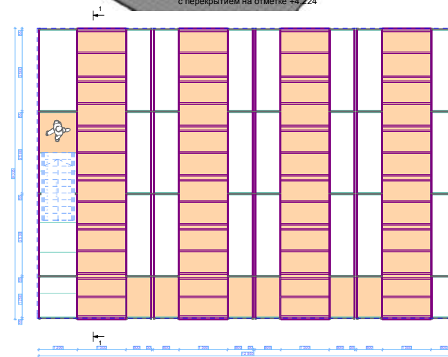
Планный расположения грузовых стеллажей с перекрытием на отметке +4,224
