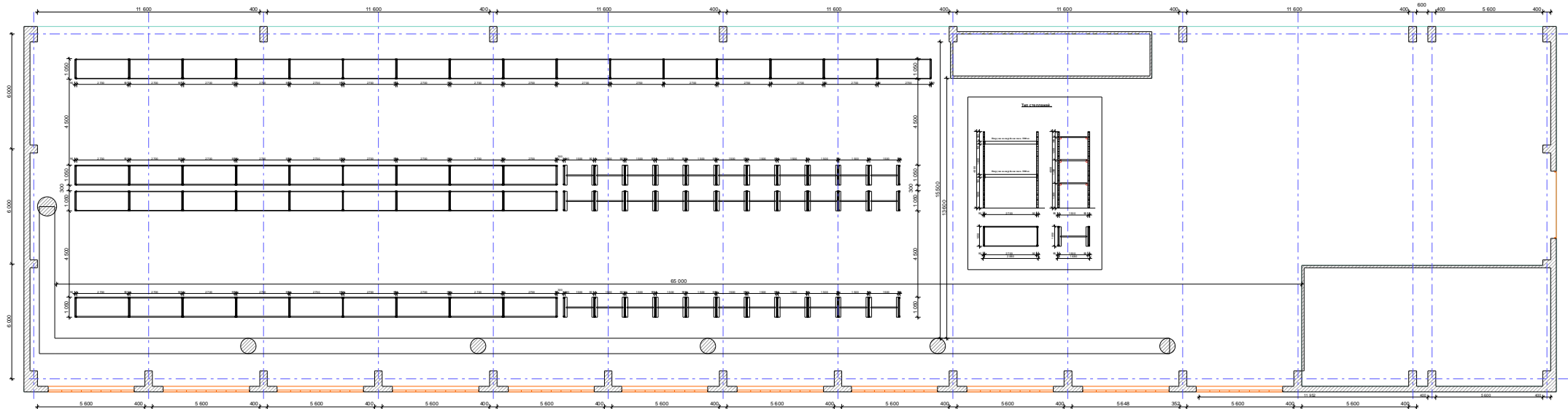
План расположения складского оборудования.
